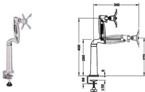
Klemmbefestigung, mittlerer Arm
