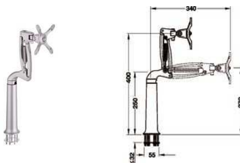
Durchsteckbefestigung, mittlerer Arm
