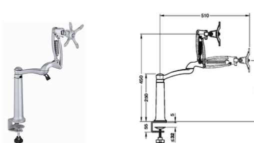
Klemmbefestigung, langer Arm
