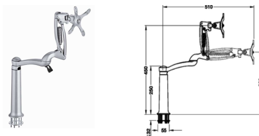
Durchsteckbefestigung, langer Arm
